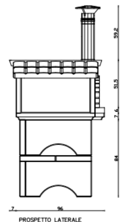
PROSPETTO LATERALE
