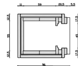
SEZIONE 1-1
