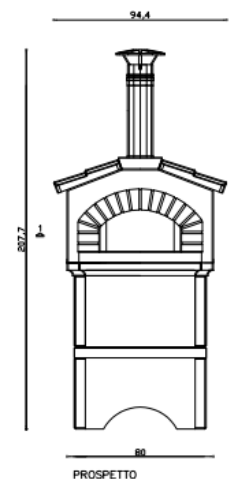
PROSPETTO
